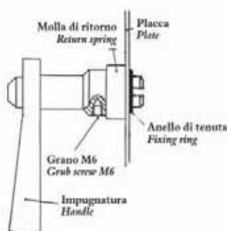
Molla di ritorno - Return spring
